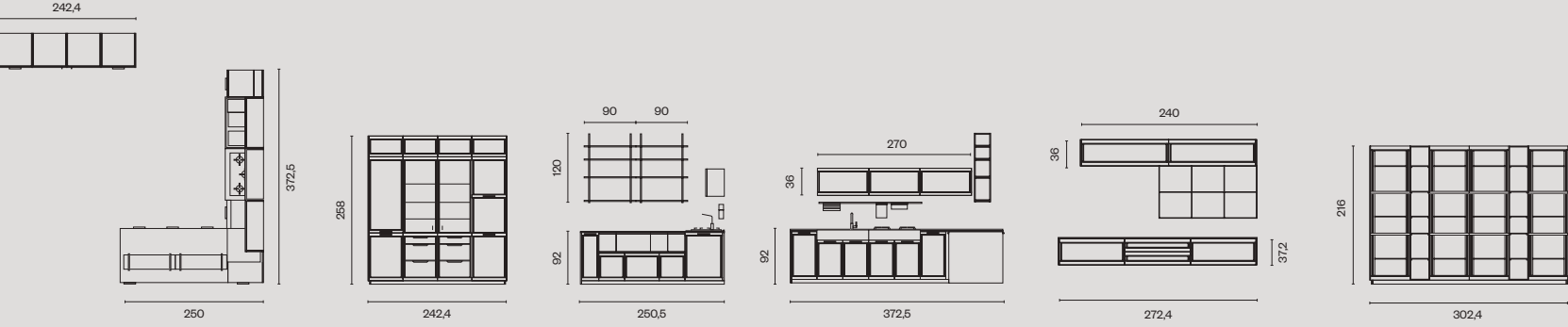
Elementi a giorno Class Alluminio verniciato rame, schienali laminato Calacatta finitura mn (opz. 6019)
