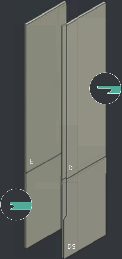
TIPO D - DS - E ANTA PER COLONNE CON PRESA VERTICALE CON E SENZA SAGOMATURA
